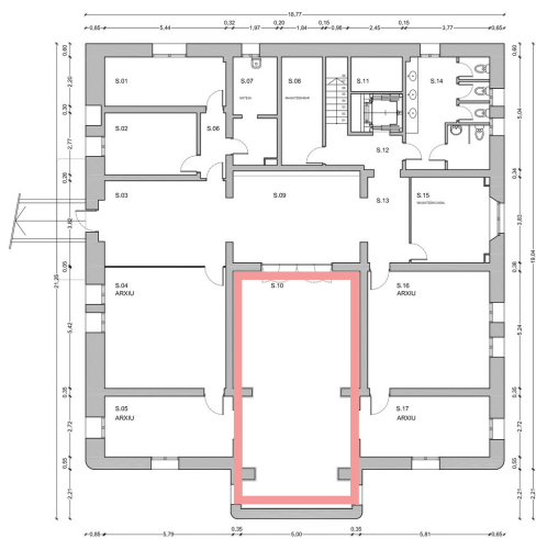
PLANTA SEMI SOTERRANI
