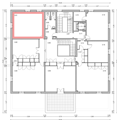
PLANTA TERCERA
