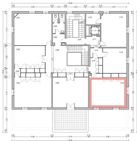
PLANTA TERCERA
