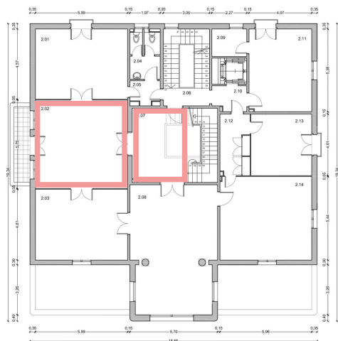
PLANTA SEGONA
